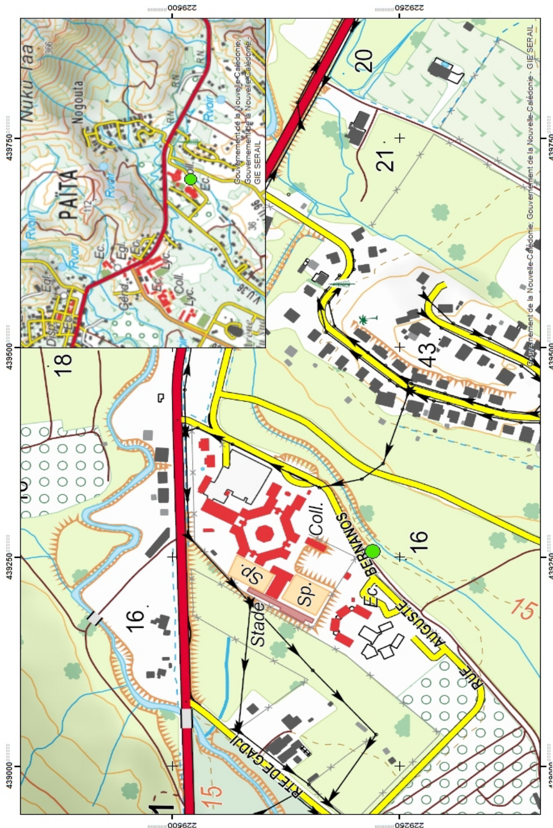
Plan de situation exutoire eaux pluviales Commune de Païta
