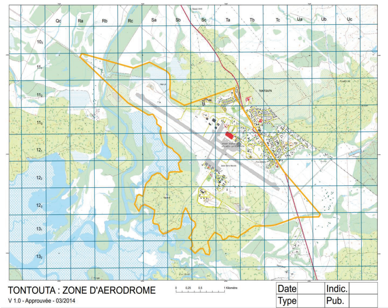
Figure 3: Zone d'aérodrome de l'aéroport de Nouméa - La Tontouta
